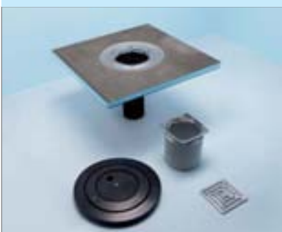
wedi Bauplatte Balco, Ablauf-Set
